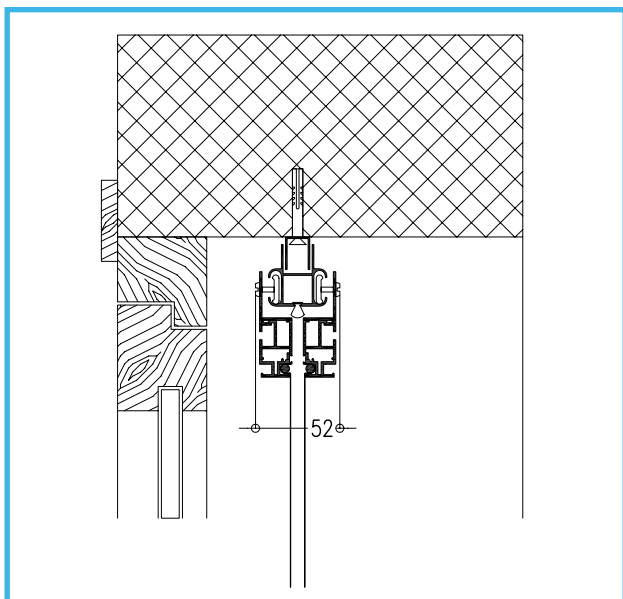
sezione verticale
