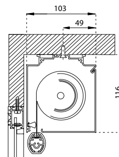
Montaggio a soffitto/parete diretto Top/front fix without bracket
