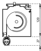
Fondale 19x23 Bottom rail 19x23
