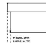
Tolleranza laterale del tessuto Fabric lateral tolerance
