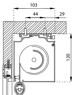
Montaggio a soffitto con supporto Top fix with bracket
