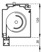
Fondale 15x20 Bottom rail 15x20
