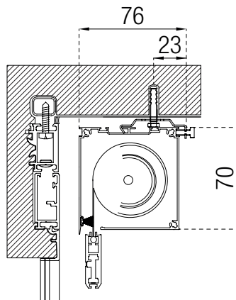
Montaggio a soffitto con supporto Ceiling installation with bracket
