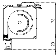
Fondale 15x20 Bottom rail 15x20
