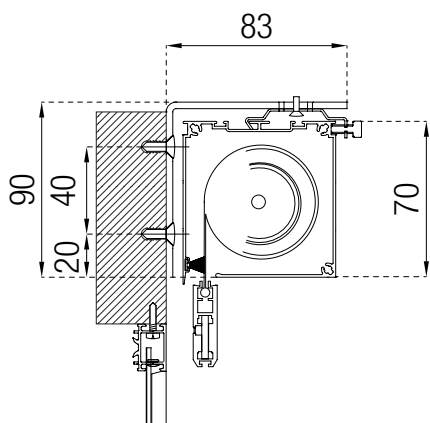
Montaggio a parete con staffa Wall installation with bracket
