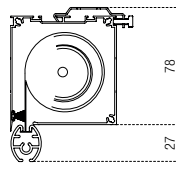
Fondale 19x23 Bottom rail 19x23
