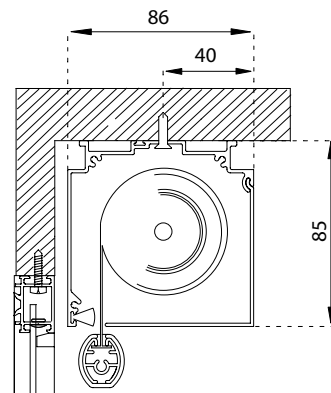
Montaggio a soffitto/parete diretto Top/front fix without bracket
