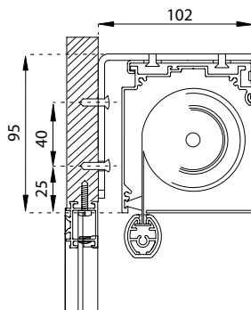
Montaggio a parete con staffa Front fix with front bracket
