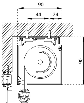
Montaggio a soffitto con supporto Top fix with bracket
