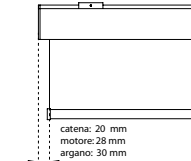
Tolleranza laterale del tessuto Fabric lateral tolerance
