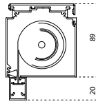
Fondale 15x20 Bottom rail 15x20
