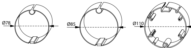
Ø78
