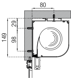
Montaggio a soffitto/parete diretto Ceiling/wall support without bracket
