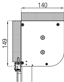
Montaggio con autoportante Self-supporting Installation
