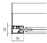
Guida Z55 Guide Z55
