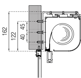
Montaggio a parete con staffa Wall installation with bracket
