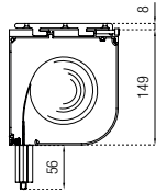
Cassonetto CT140 Cassette CT140
