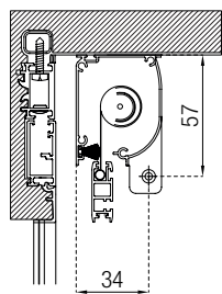
Cassonetto C40 con autoportante Self-supporting cassette C40
