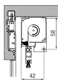
Cassonetto C 46 con autoportante Self-supporting cassette C46
