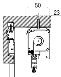
Cassonetto C 46 con supporto Cassette C46 with brackets
