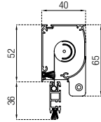
Cassonetto C40 Cassette C40
