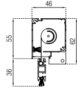
Cassonetto C46 Cassette C46
