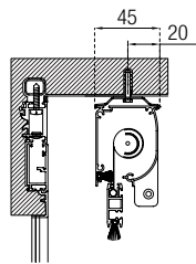
Cassonetto C 40 con supporto Cassette C40 with brackets
