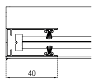
Guida 22x40 Guide 22x40
