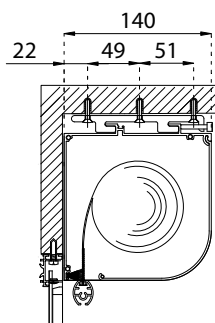
Montaggio a soffitto con supporto Ceiling mounted with bracket
