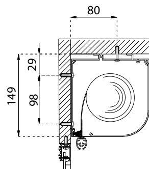
Montaggio a parete/soffitto diretto Directly wall-ceiling mounted
